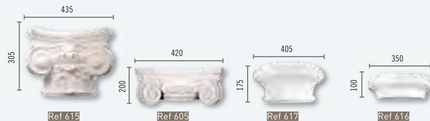
Chapiteaux Kapitelen
