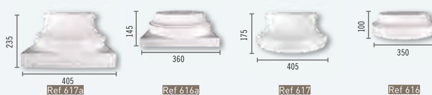
Socles Voetstuk
